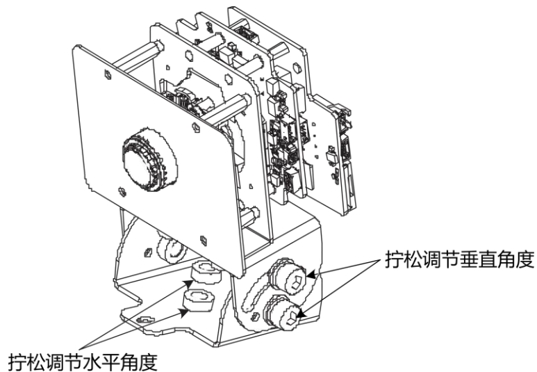
图4-2 调整镜头位置
