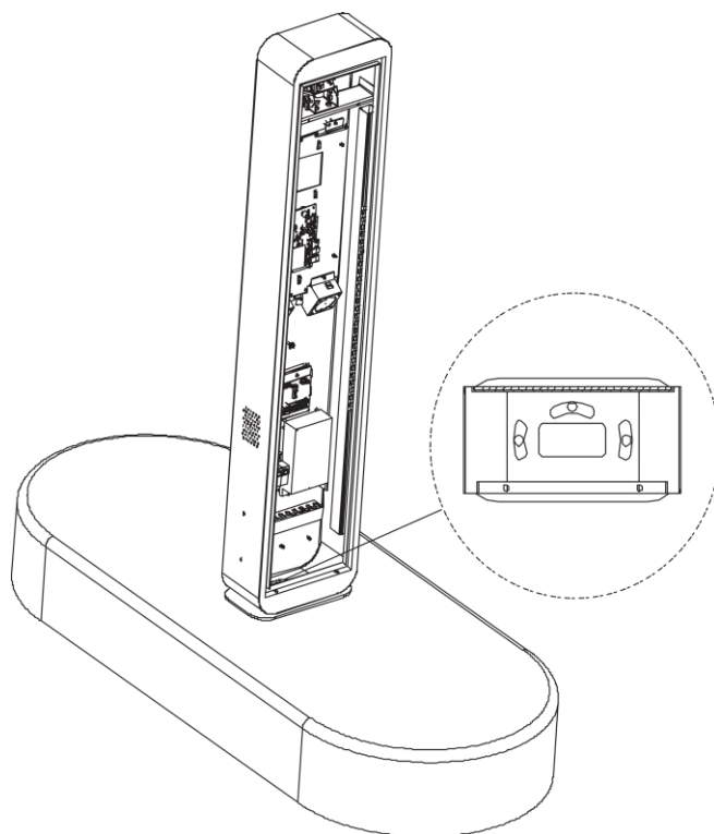
图2-4 固定机身
