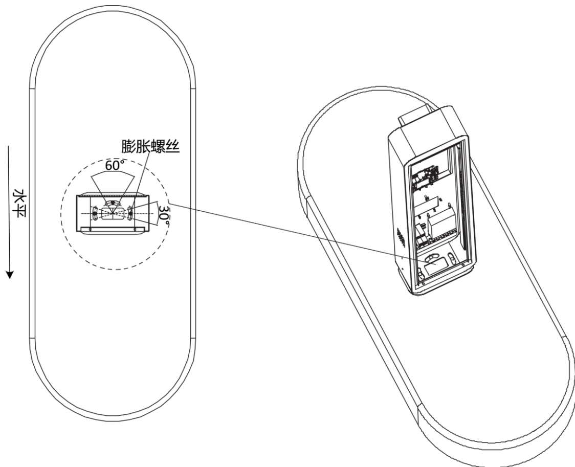
图4-1 调整机箱角度
