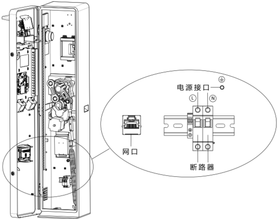
图2-5 线缆接口
