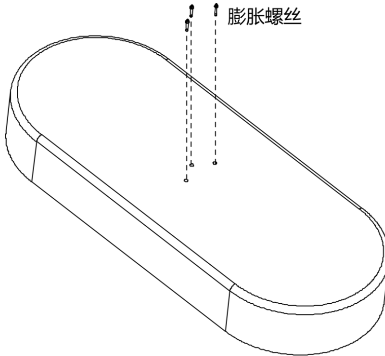
图2-2 安装膨胀螺丝
