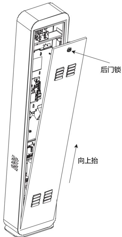
图2-3 打开机箱后门
