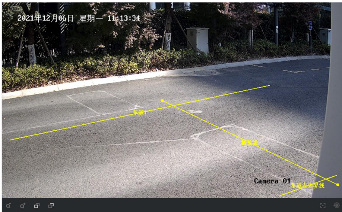
图4-4 车道线和触发线
