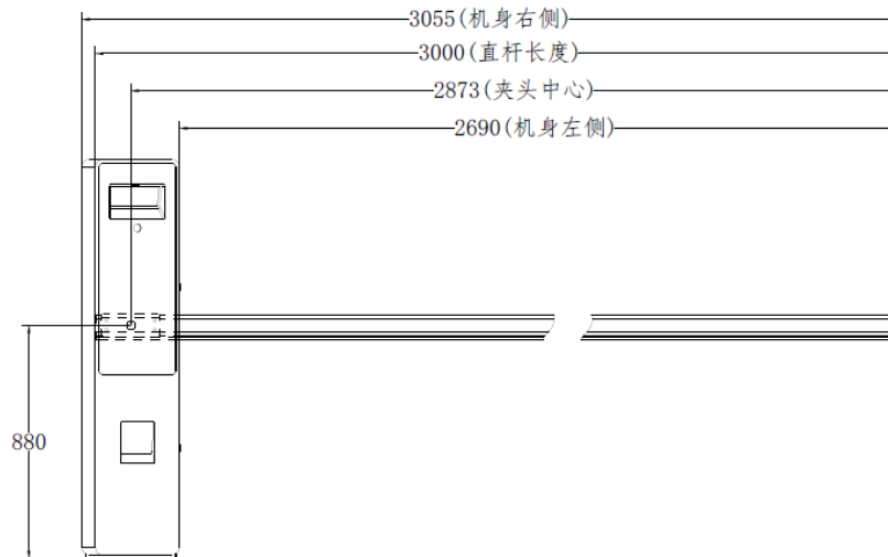
3米横杆（左侧道闸对称，尺寸相同）
