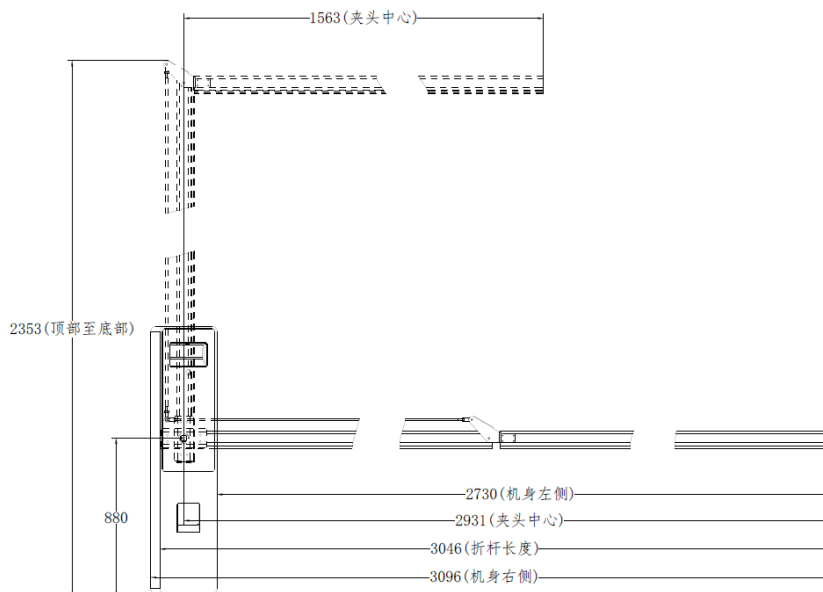
1.5+1.5米曲臂杆 (左侧对称, 尺寸相同)
