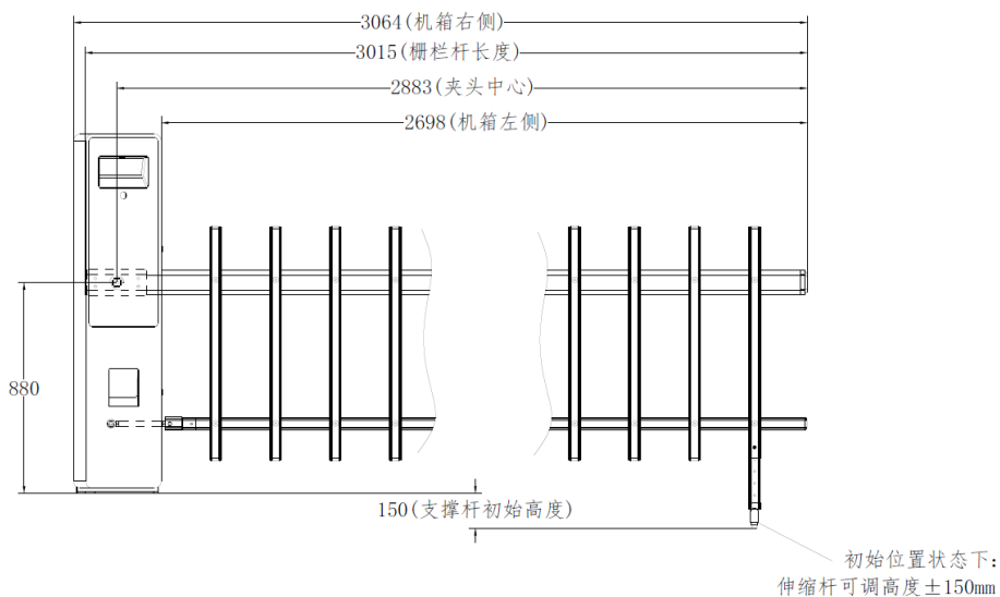
3米栅栏杆 (左侧对称, 尺寸相同)
